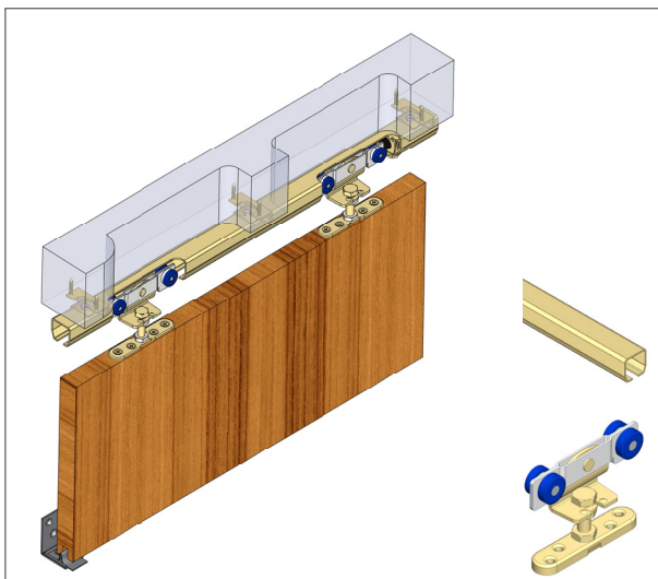
Schiebetür-Set mit Stahl-Laufschiene | NIKO Profil 21. - bis zu 75 kg
