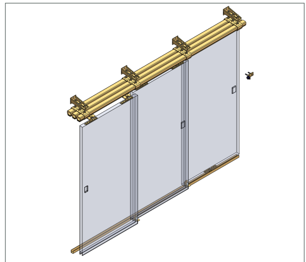
Schiebetor dreiflügelig
