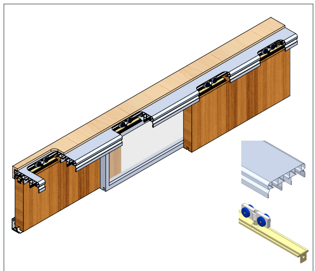
Schiebetür-Set mit Aluminium-Laufschiene | NIKO Profil 04. - bis zu 60 kg
