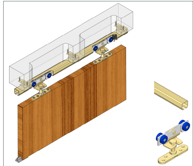
Schiebetür-Set mit Stahl-Laufschiene | NIKO Profil 12. - bis zu 60 kg
