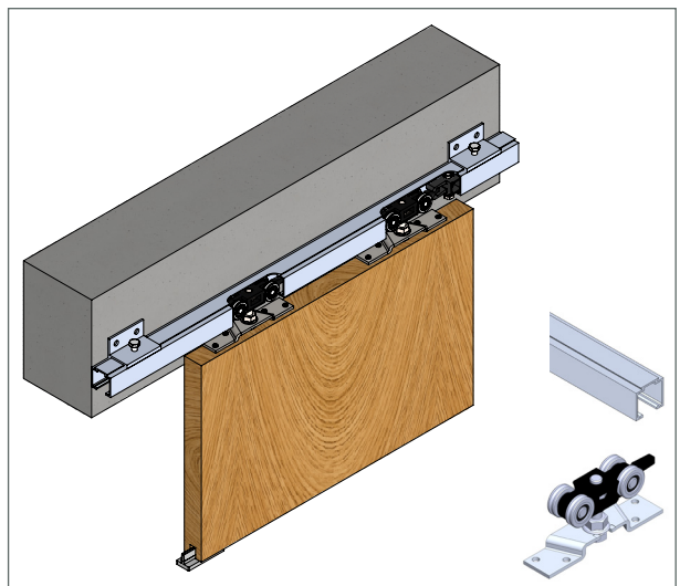
Schiebetür-Set mit Aluminium-Laufschiene | NIKO Profil 80. - bis zu 80 kg
