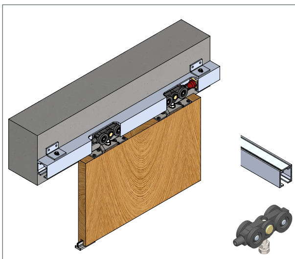
Schiebetür-Set mit Aluminium-Laufschiene | NIKO Profil 84. - bis zu 125 kg
