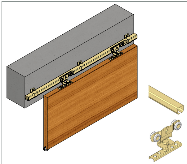
Schiebetür-Set mit Stahl-Laufschiene | NIKO Profil 11. - bis zu 13kg
