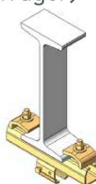
.B36 Vertikal zum Träger
