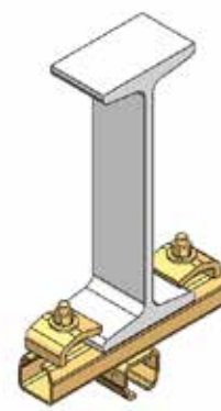
.B35 Parallel zum Träger
