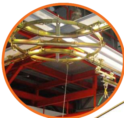
.A43 Drehscheiben- weiche
